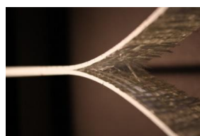
Abb.2: Mode I Rissöffnung.
